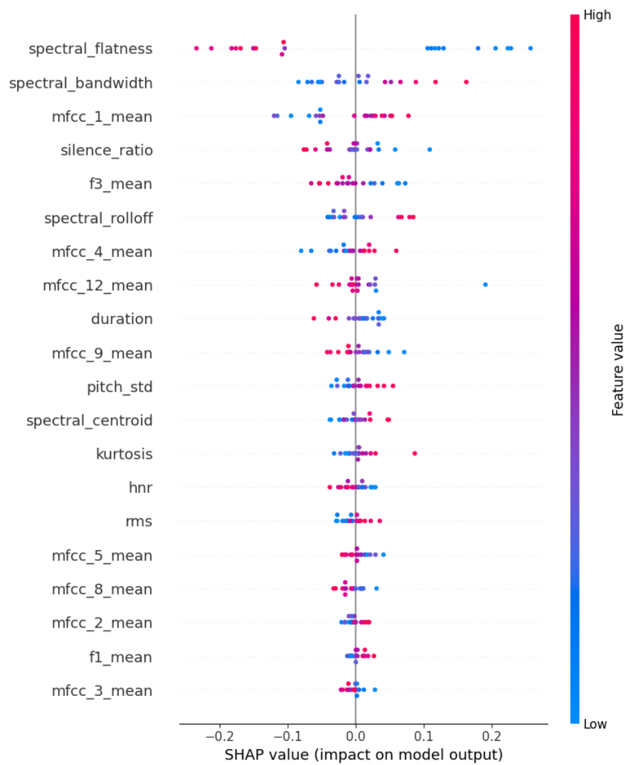
Figura 35: Explicación global con SHAP
