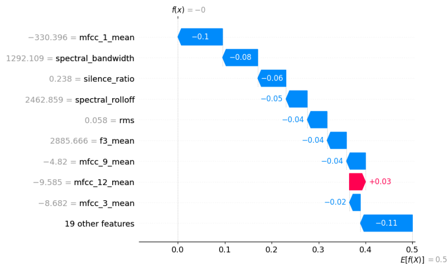
Figura 36: Explicación local con SHAP tras quitar spectral flatness
