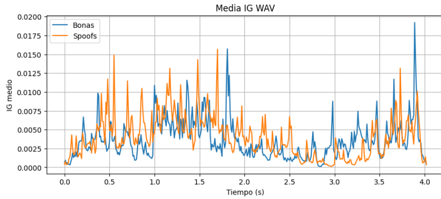
Figura 50: Importancia temporal al aplicar IG sobre onda de audio cruda.
