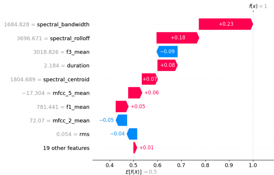
Figura 37: Explicación local con SHAP tras quitar spectral flatness
