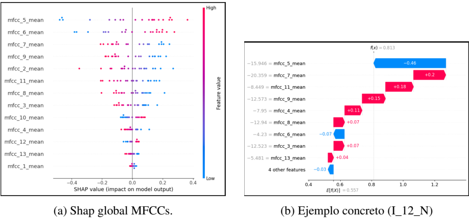
Figura 56: Influencia de características espectrales en Wav2Vec2
