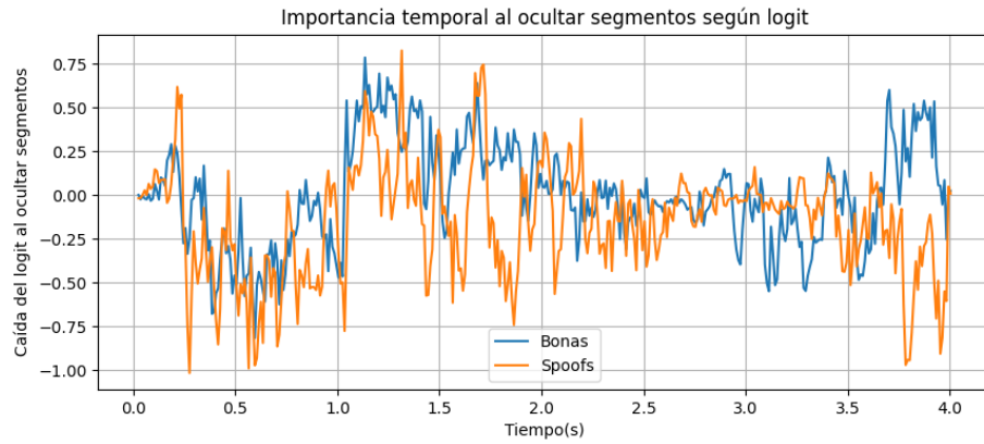
Figura 43: Resultados de “logit” de la ocultación temporal en AASIST.
