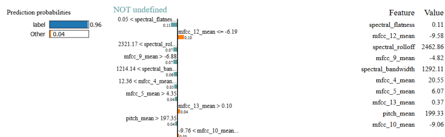
Figura 40: Explicación local con LIME
