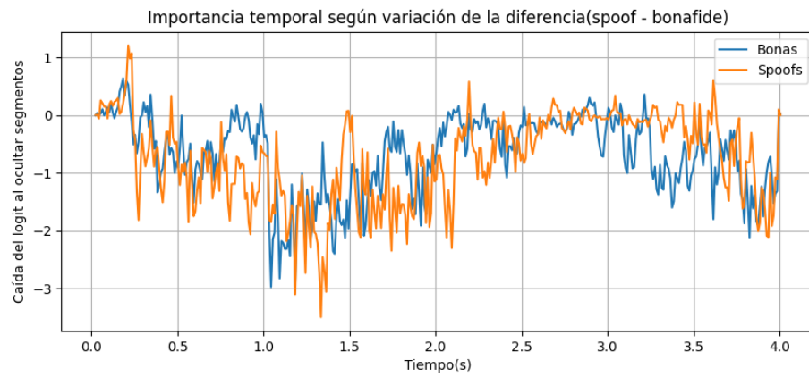
Figura 44: Resultados de margen de la ocultación temporal en AASIST.
