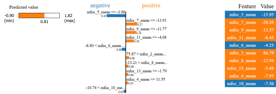
Figura 60: Explicación local mfccs Lime.
