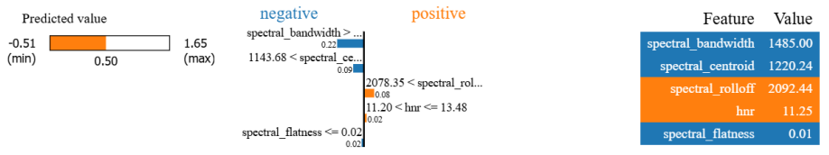
Figura 57: Explicación local espectrales Lime.
